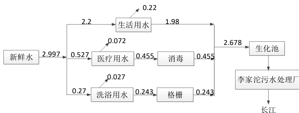
图 3.6-1 本项目水平衡图 m 3 /d
